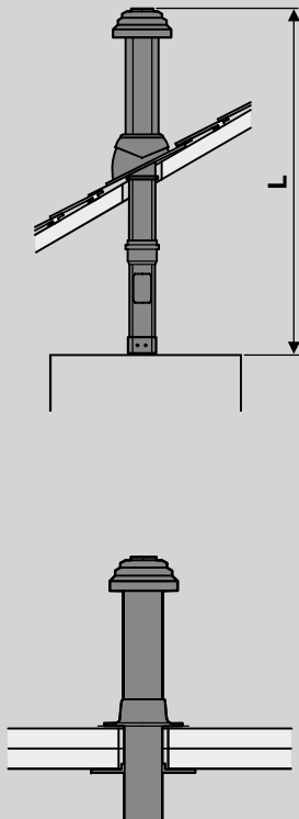
Instalación C33x DN 60/100 y 80/125
