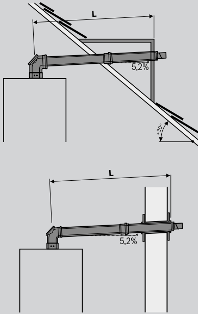
Instalación C33x DN 60/100 y 80/125
